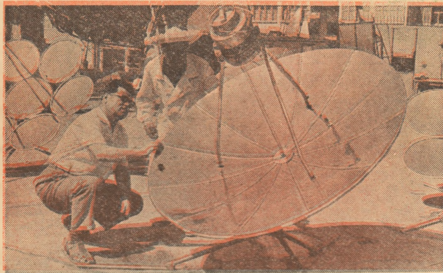
Bucătărie solară — pentru încălzit apă, preparat mâncare etc. Principalul element al instalației este un reflector parabolic, care concentrează razele solare. O uzină uzbekă urmează să producă anual 25 000 bucătării solare
