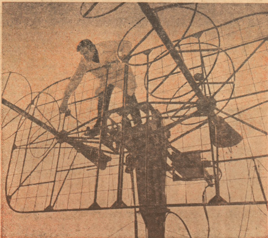
Antena care recepționează semnale transmise de sateliții meteorologici ai Pămîntului (la stația aerologică din Tbilisi).
