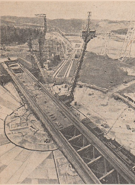
La Krasnoiarsk, pe Enisei se construiește un lift pentru navele fluviale menit să înlocuiască ecluzele
